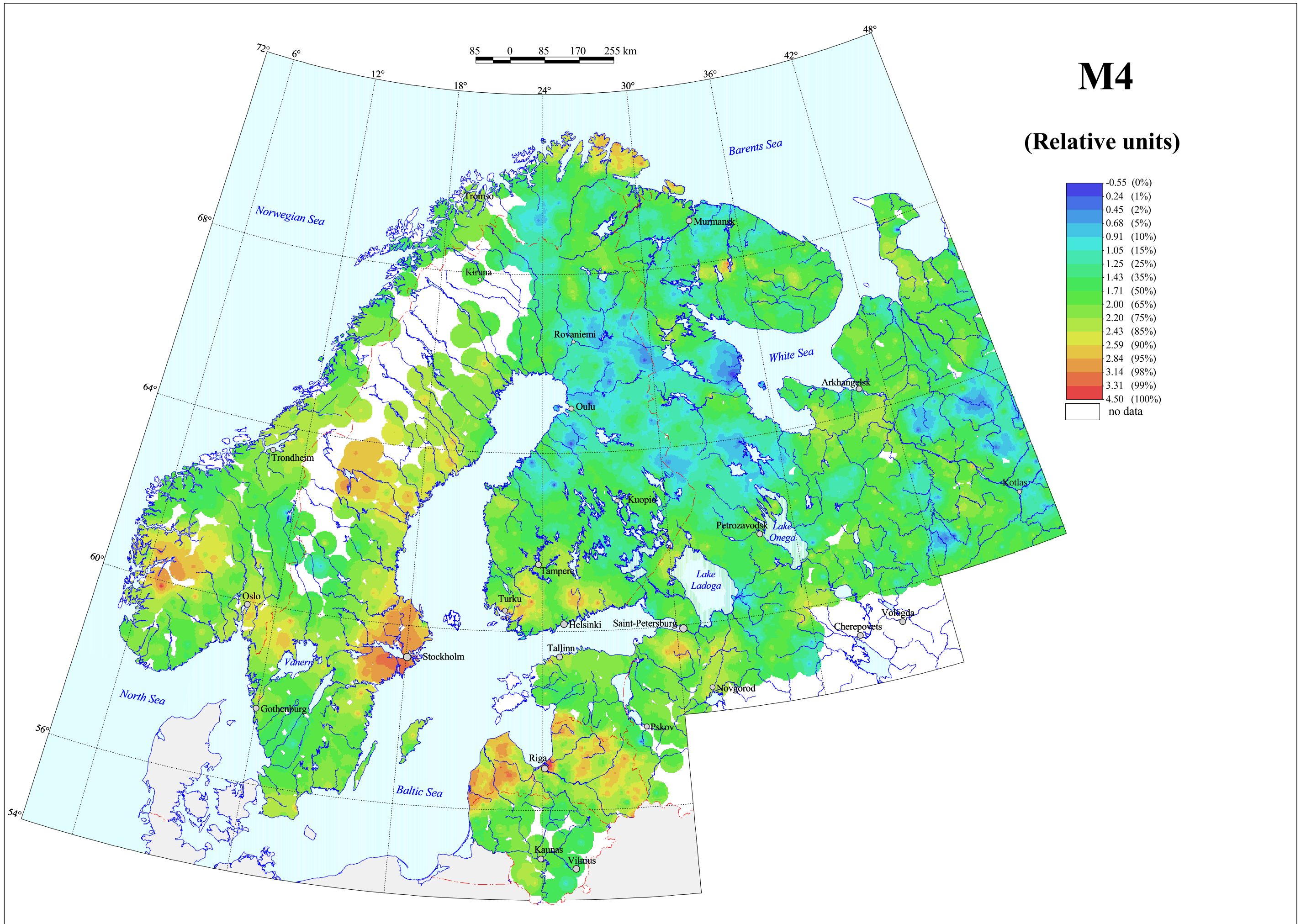
M4 (Pb, Zn) in C-horizon, Grain Size <2 mm, Aqua regia Extraction
